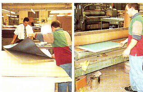
Laminados y chapa de madera sobre madera (Puertas)
