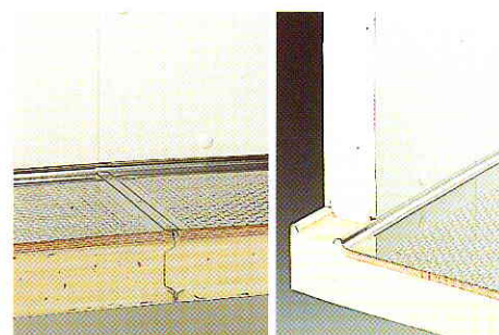
Espumas rígidas a metales pintados (Almacenes y salas refrigeradas: paneles tipo "Sandwich")
